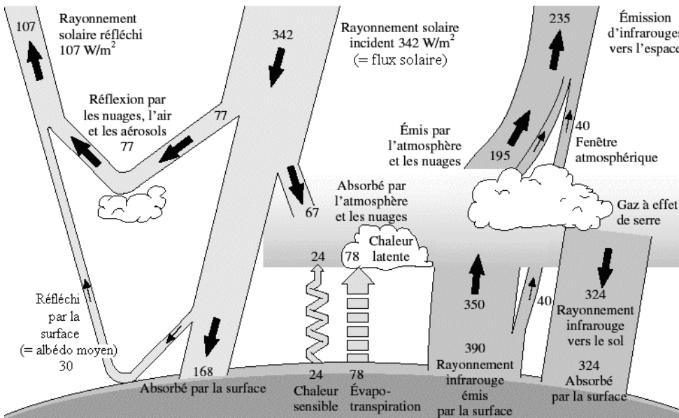
Bilan radiatif (équilibré) de la Terre.
